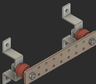
Barre de mise à la terre Grounding bar
